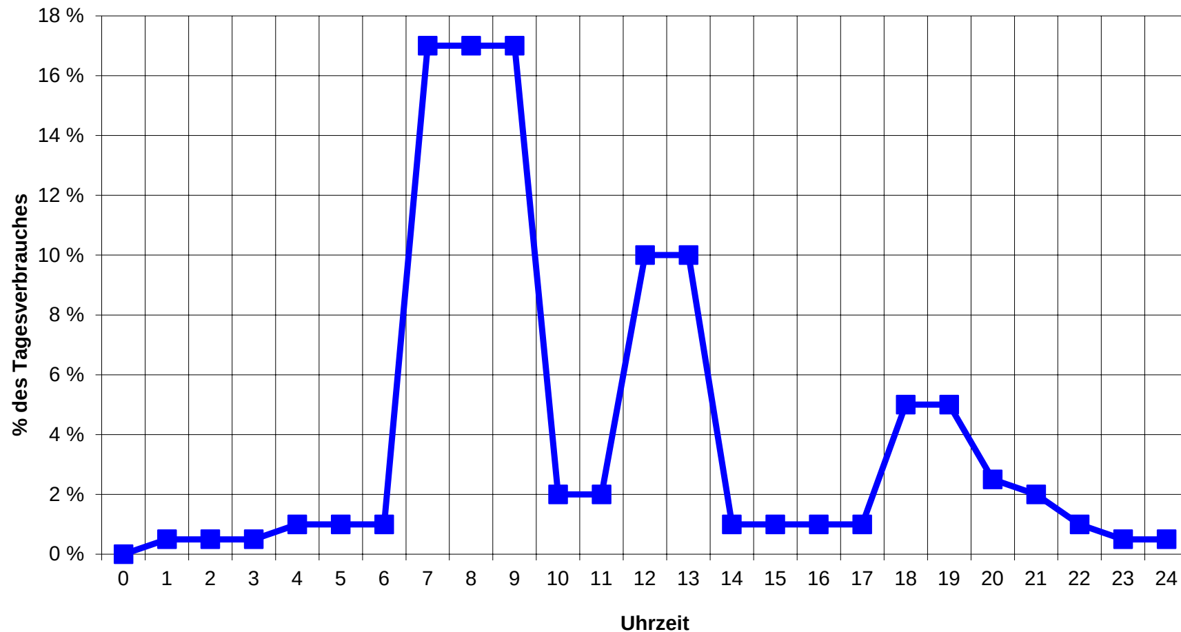
Verbrauchscharakteristik
