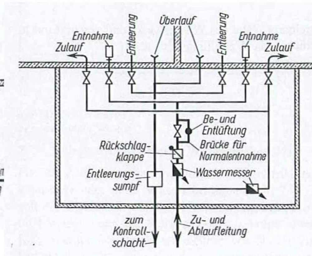
Rohrschema Gegenbehälter
