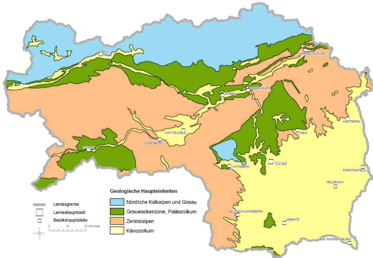
Abbildung 8: Geologische Übersichtskarte der Steiermark, Quelle: www.schulatlas.at
