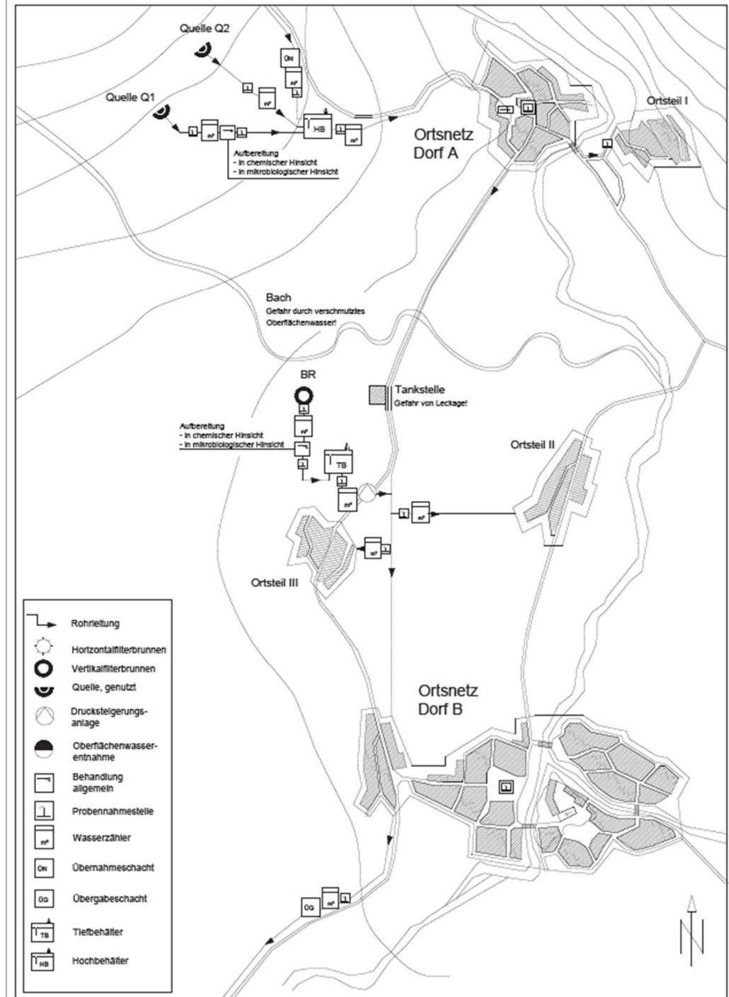
Abb. 1 Beispiel eines Übersichtslageplans
